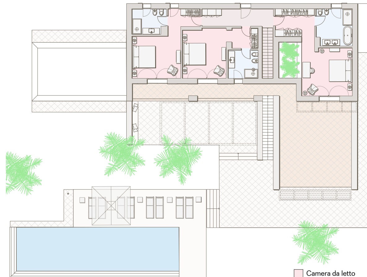
PRIMO PIANO
